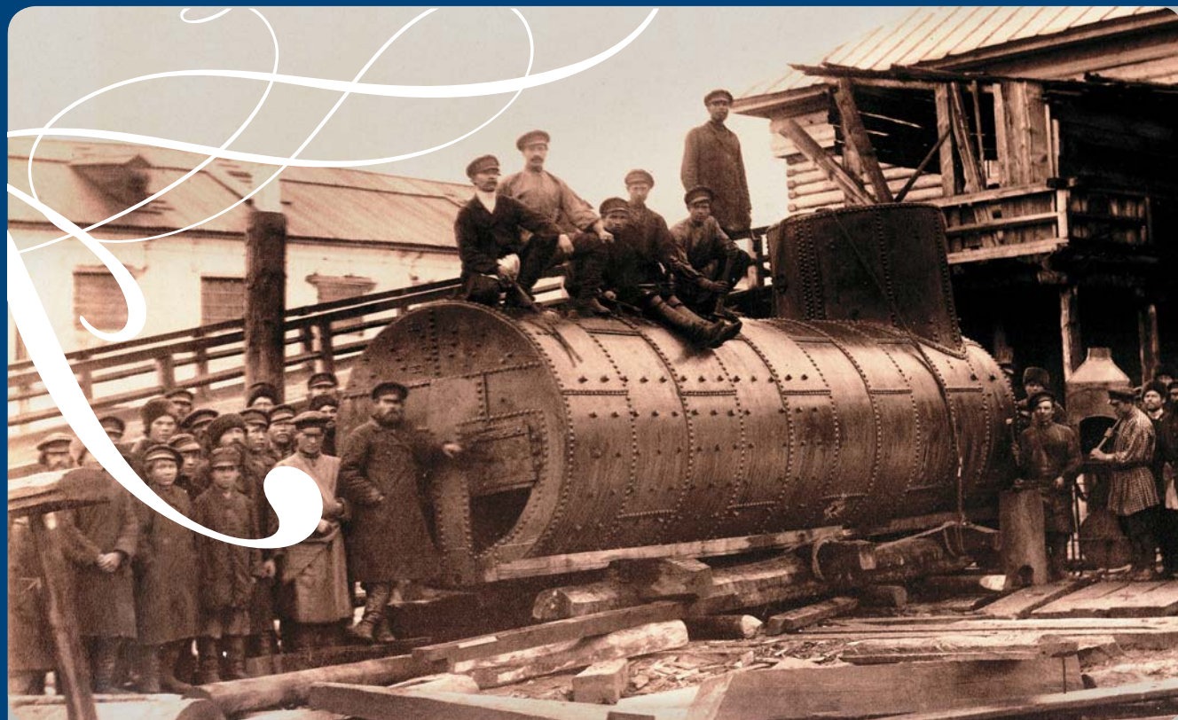
Винокуренный завод в старинном селе Тельма под Иркутском. Новый паровик. Из альбома фабрично-заводской промышленности Иркутской губернии 1895—1896 гг., изд. В. Ап. Белоголового
