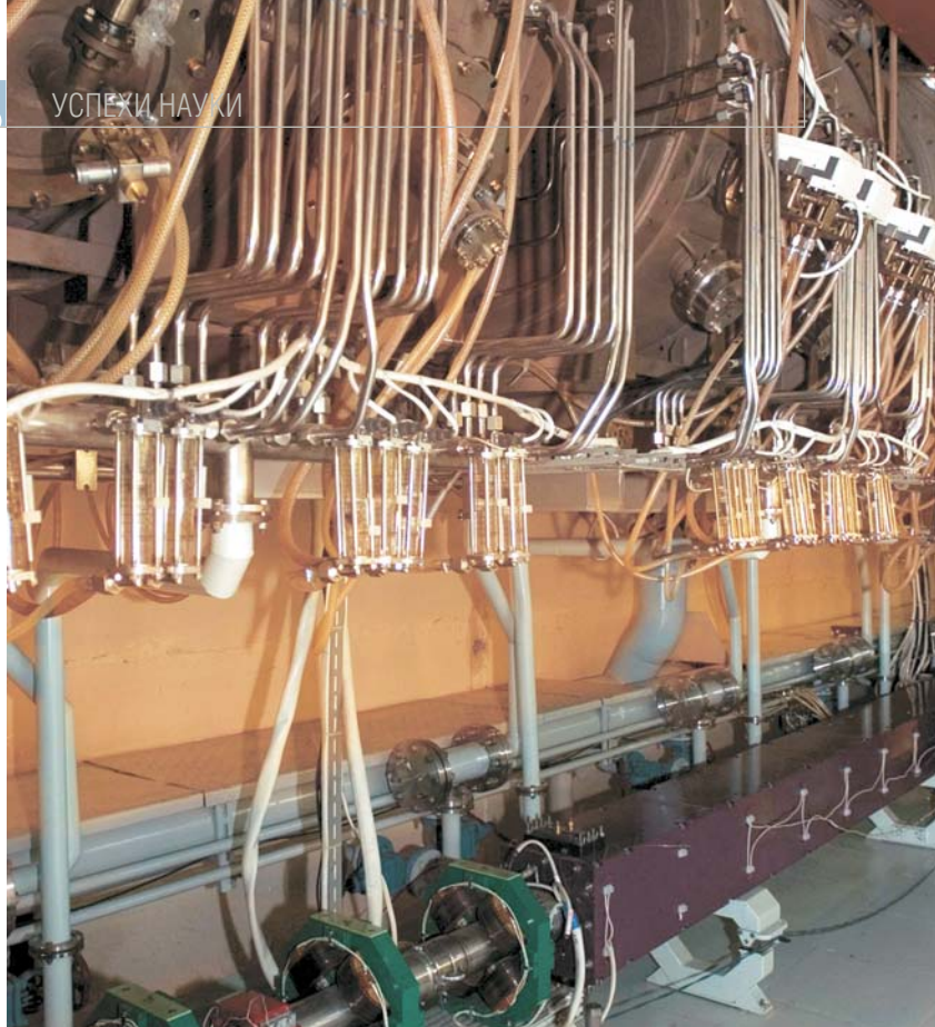
Первая очередь установки с ЛСЭ, запущенная в апреле 2003 г., в отличие от полномасштабного варианта имеет единственный канал транспортировки электронов
