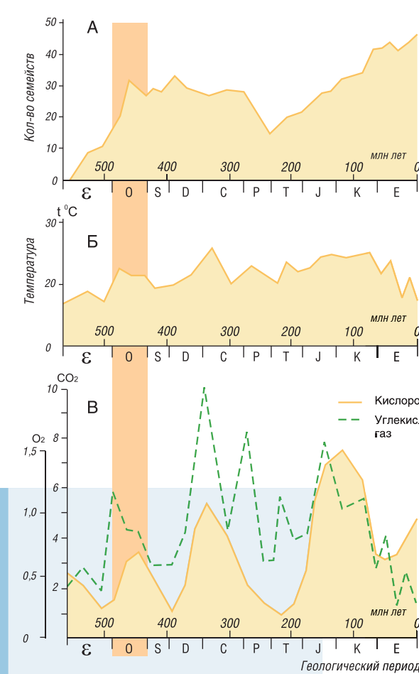
Динамика биоразнообразия (А), теплового режима (Б), и относительных масс (по сравнению с современными) углекислого газа и кислорода (В) (по Будыко и др., 1985)
