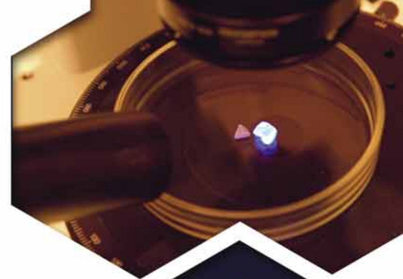
Октаэдрический кристалл алмаза в обычном, поляризованном свете и ультрафиолетовом свете
