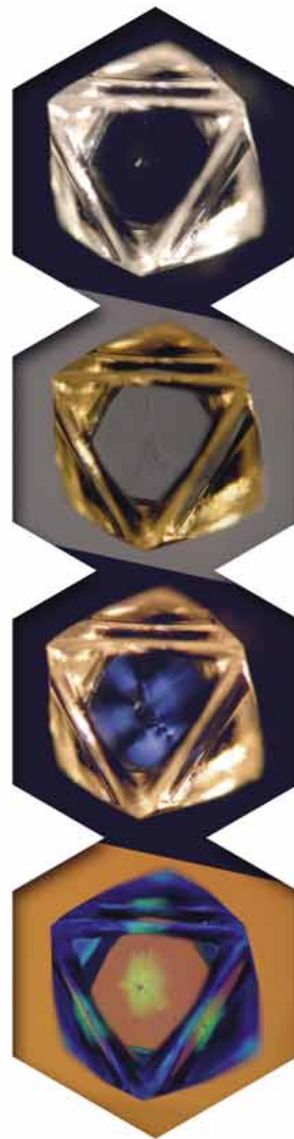
Октаэдрический кристалл алмаза в обычном, поляризованном свете и ультрафиолетовом свете
