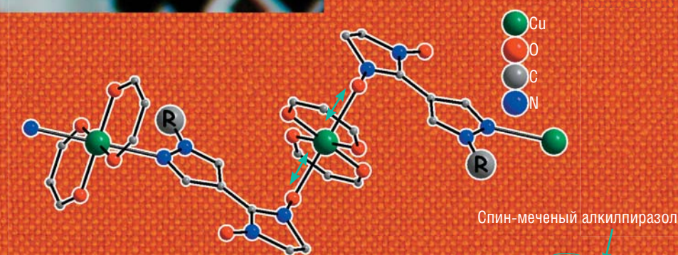
Фрагменты полимерной цепи в \text{Cu}(\text{hfac})_2\text{L}^{\text{R}}
