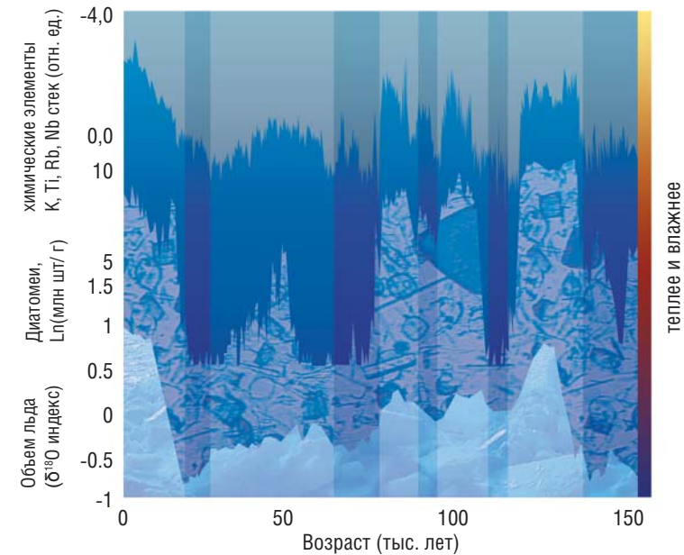
Результаты сканирования колонки осадков оз. Байкал длиной более 7 м с разрешением 1 мм (временное разрешение около 20 лет). На верхнем графике показан усредненный профиль кластогенных элементов, на среднем — содержание биогенного кремнезема (створки диатомовых водорослей) в осадках; на нижнем — объем глобальных ледовых щитов
